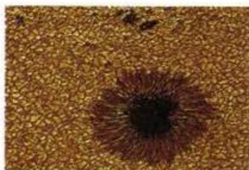
Рис. 189. Гранулы и пятно в фотосфере Солнца
